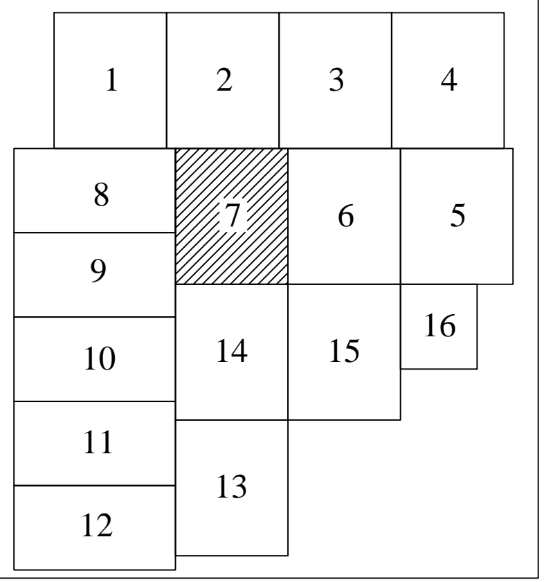
SCHEMA DE RACORDARE A PLANSELOR
